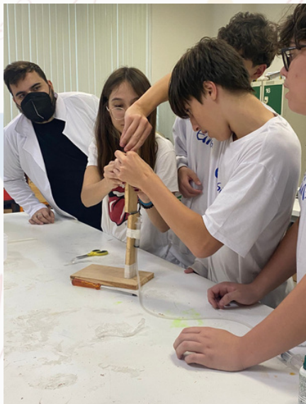
Projeto Guindaste Hidráulico (Alunos construindo um Guindaste Hidráulico funcional com madeiras e seringas).
